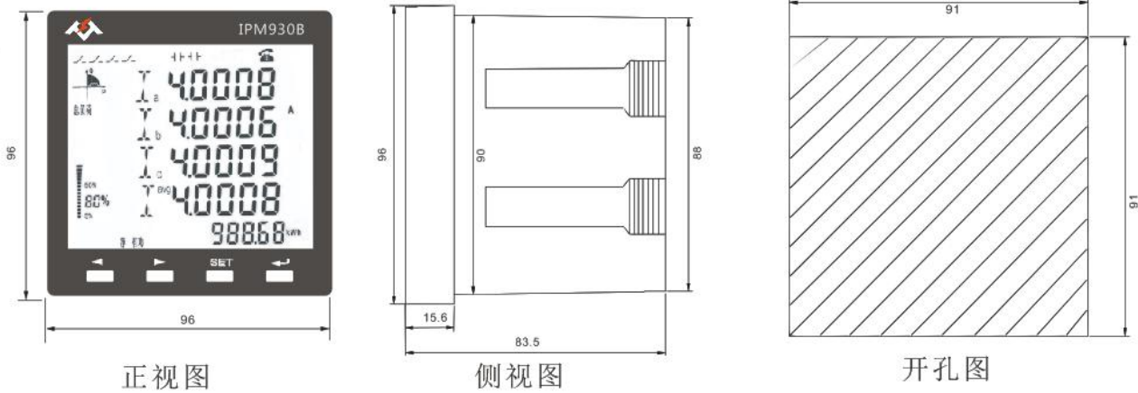
图 3-2 结构图
