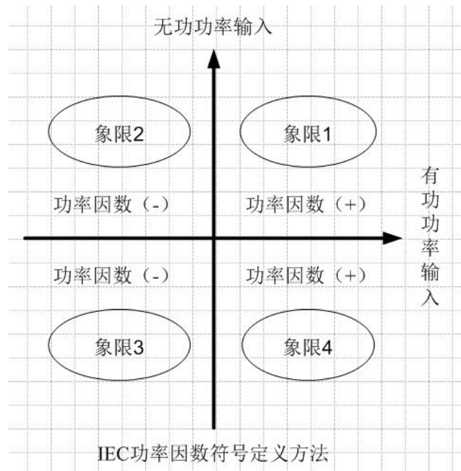
图 5-2 功率因数的定义方法
